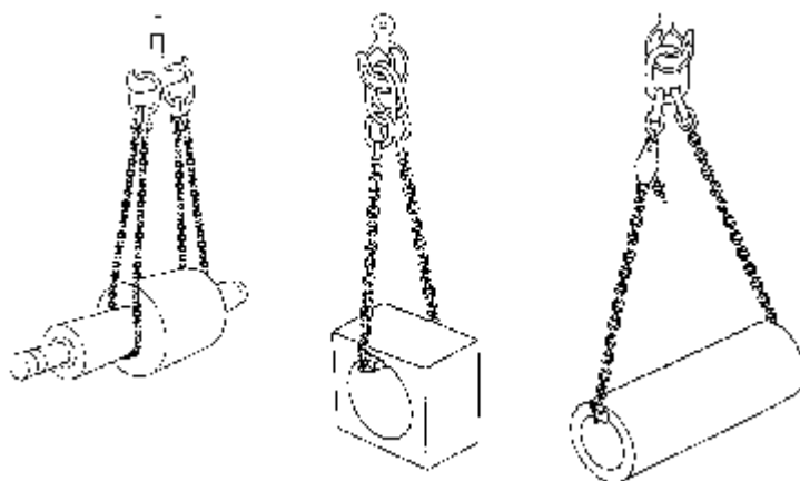
Obrázek 4 : Vázání podvlečením
