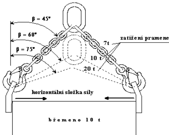
Obrázek 1 : Změna zatížení v prameni vázacího řetězu v závislosti na úhlu pramene ke svislici pro břemeno 10t
