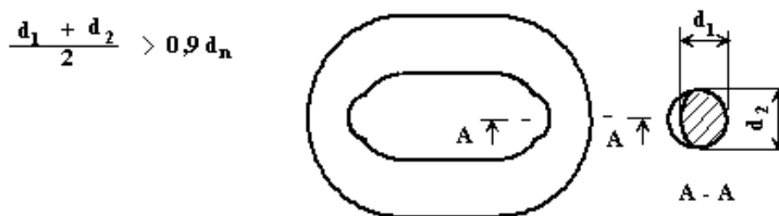
Obrázek 10 : opotřebenění mezi články
