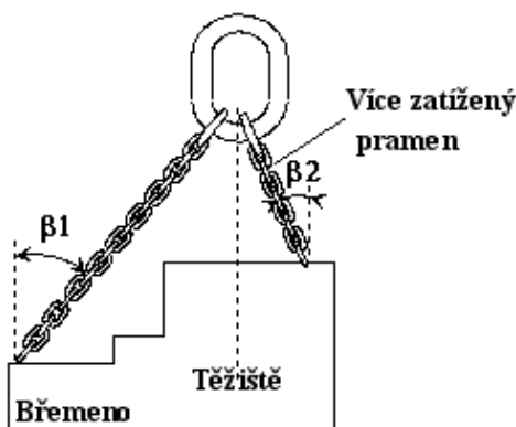
Obrázek 9 : nesymetrické zatížení
