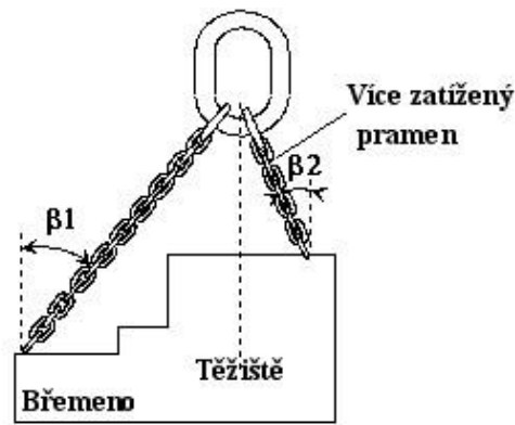
Obrázek 9 : nesymetrické zatížení
