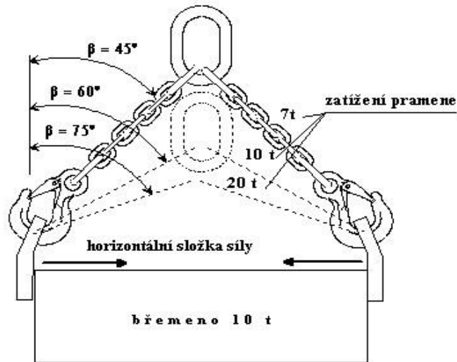
Obrázek 1 : Změna zatížení v pramenech vázacího řetězu v závislosti na úhlu pramene ke svislici pro břemeno 10t
