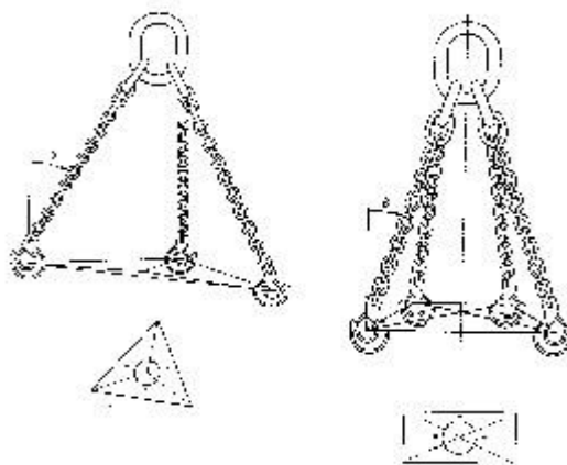
Obrázek 8 : Vícepamenné vázací řetězy – rozdělení břemene
