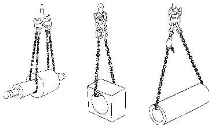
Obrázek 4 : Vázání podvlečením
